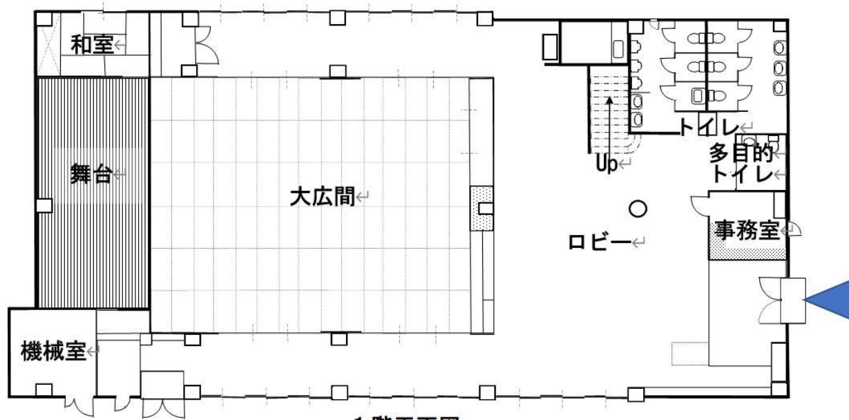
1階平面図
